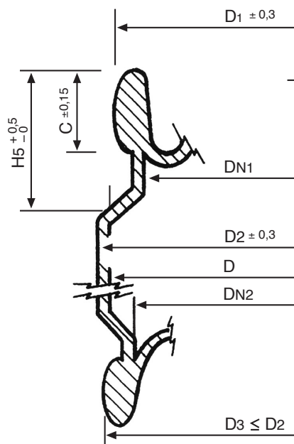
SEZ. A-A
